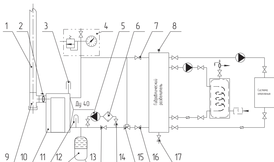
в) закрытая система с принудительной циркуляцией через гидравлический разделитель
